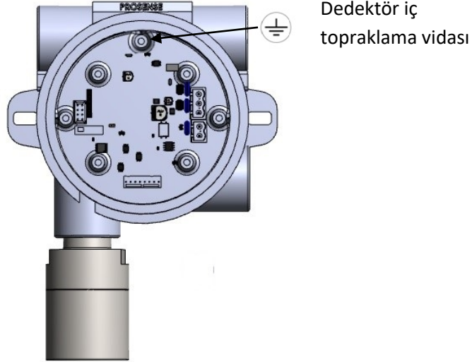
Diagram 9: Dedektör içi topraklama vidası
