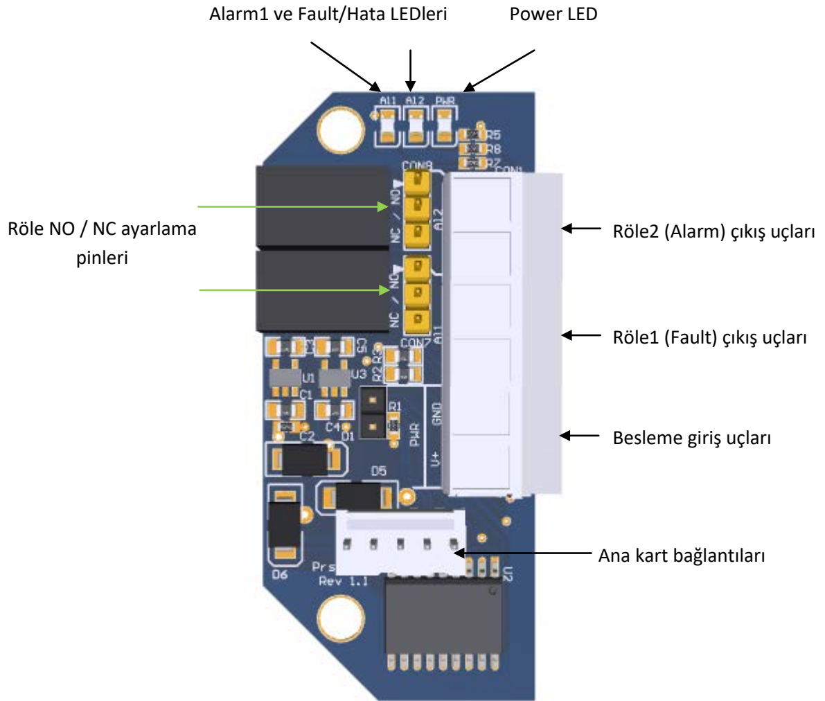
Diagram 9: Röle kartı ve bağlantılar
