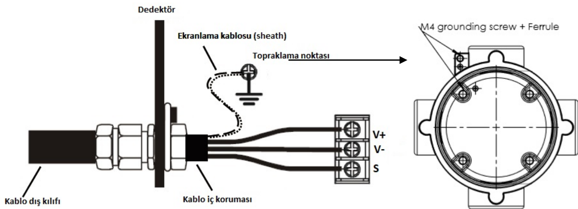
Diagram 6: Topraklama örneği
