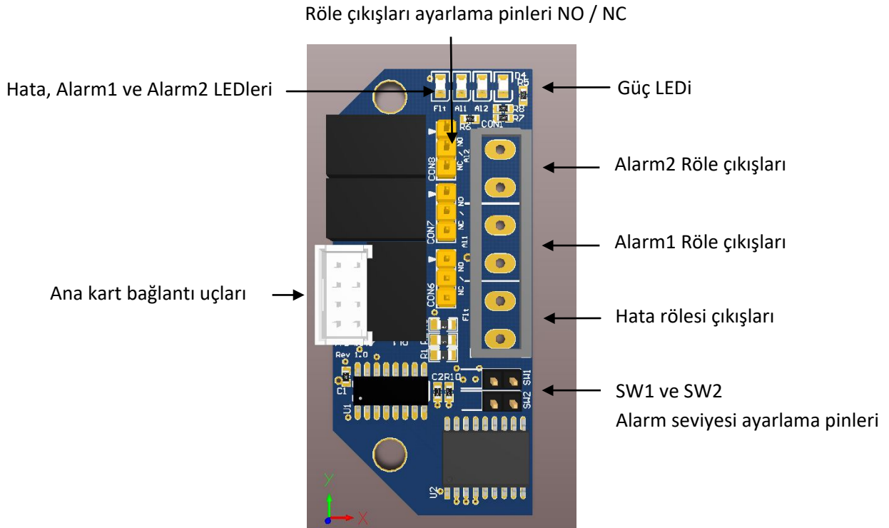
Diagram 11: Röle Modülü
