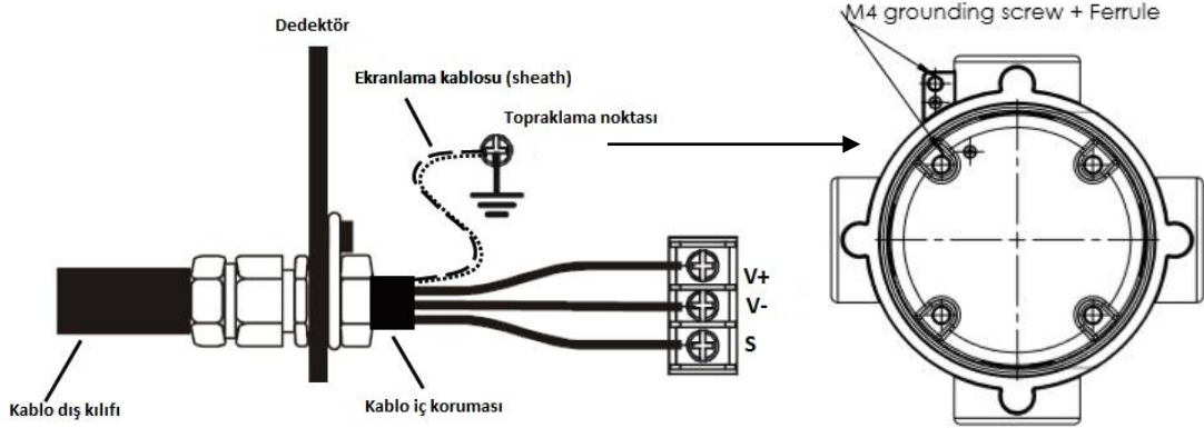
Diagram 6: Topraklama örneği
