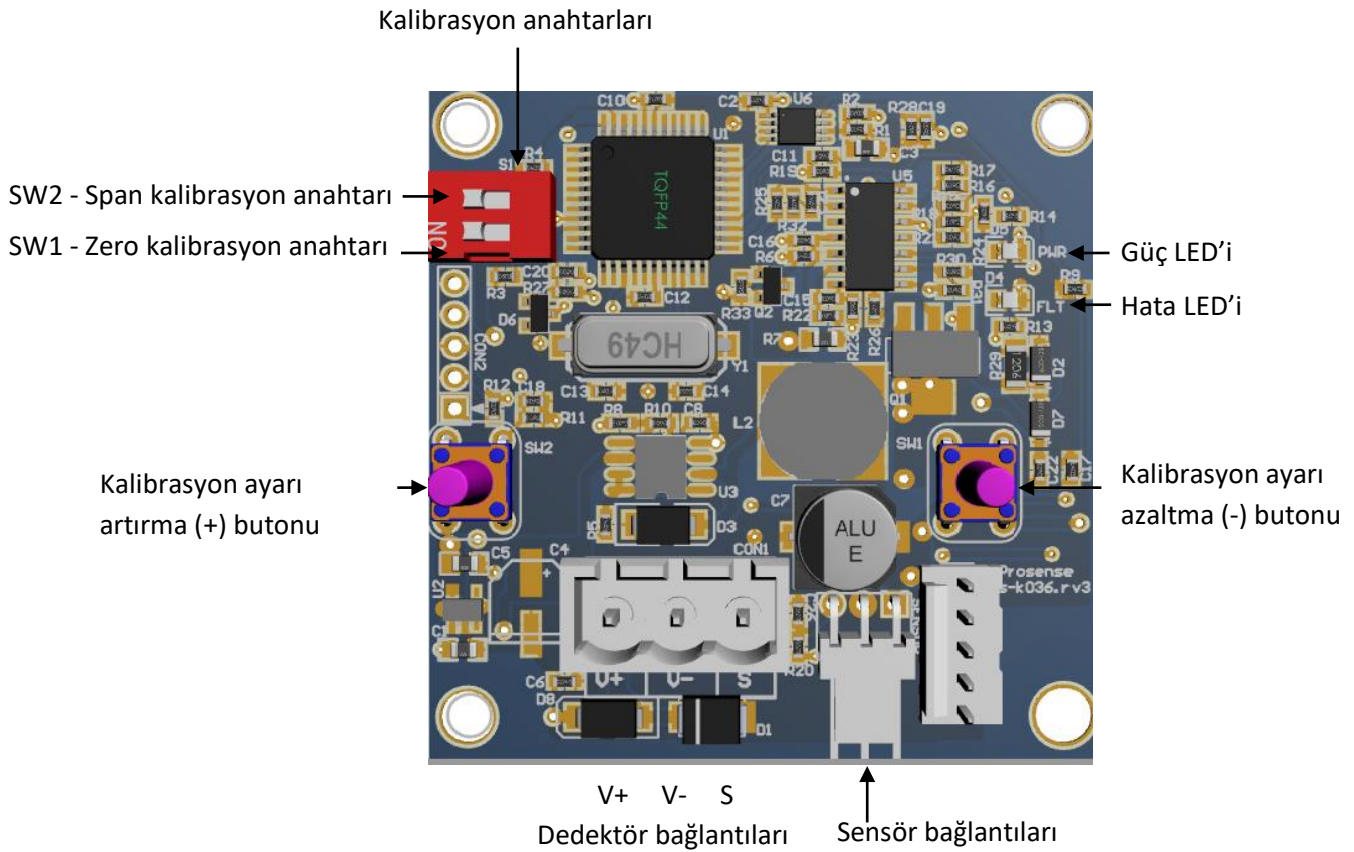
Diyagram 8: Dedektör ana kartı ve bağlantıları
