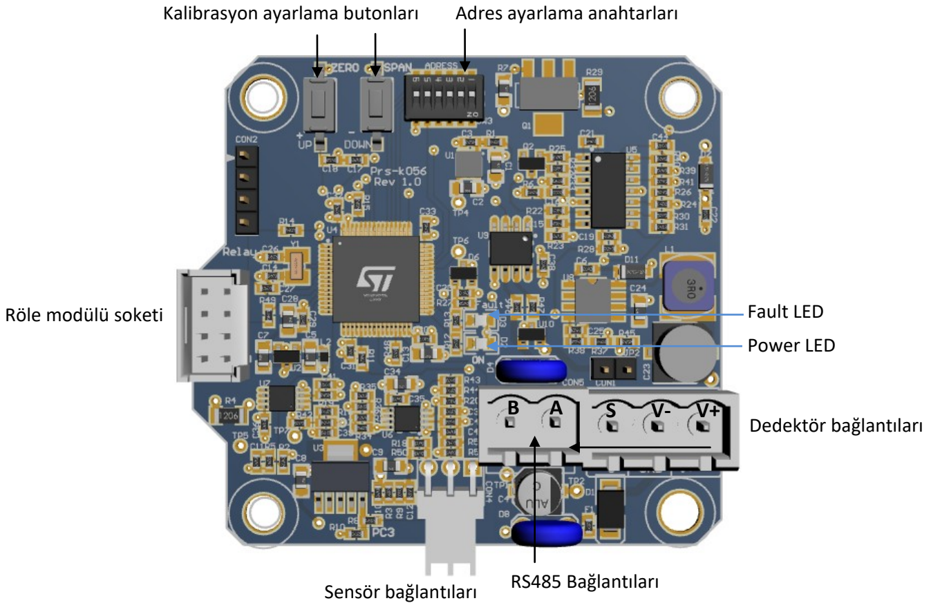
Diagram 7: Dedektör ana kartı ve bağlantıları
