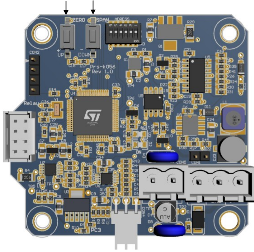
Diagram 10: Kalibrasyon butonları
