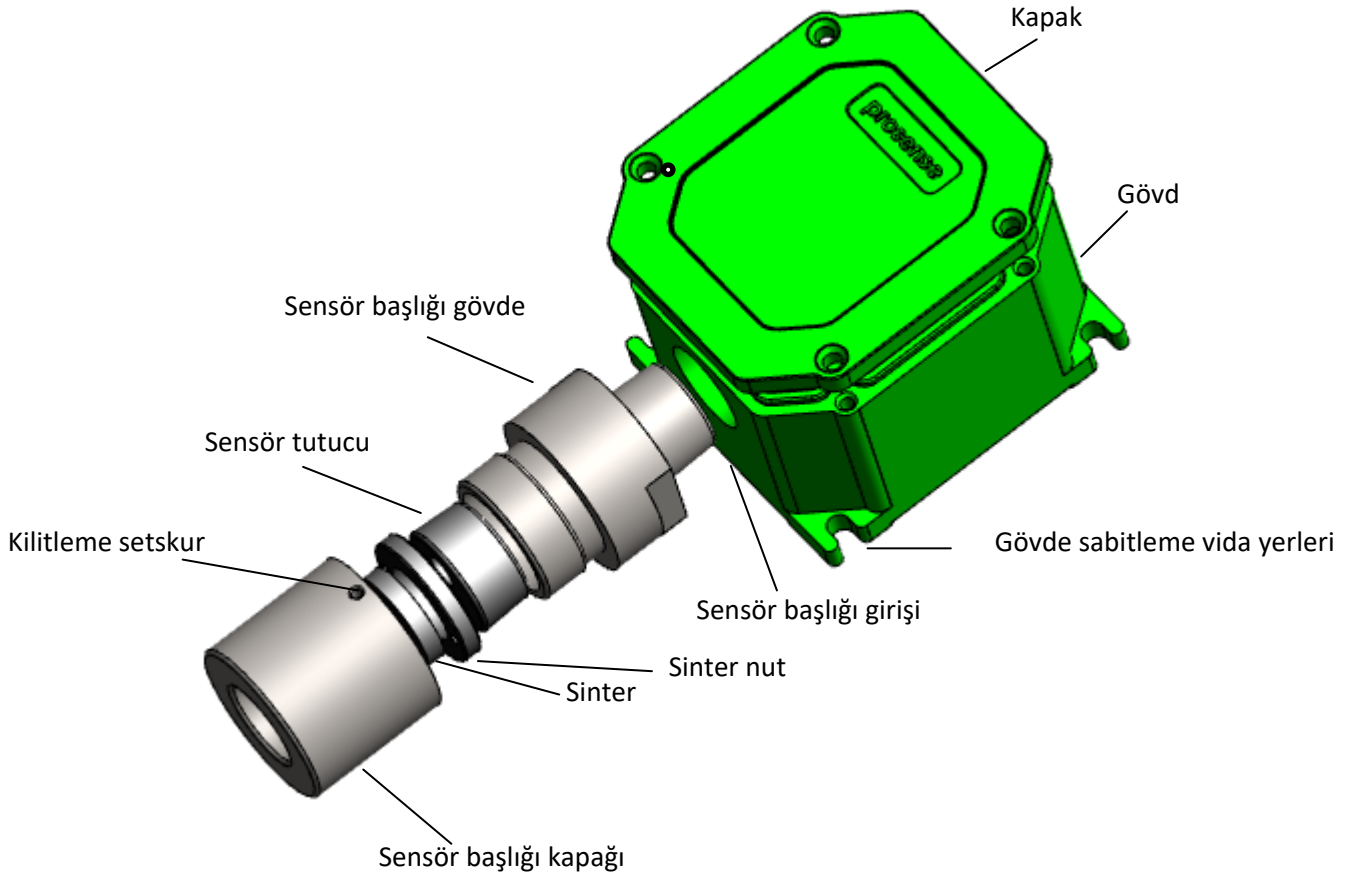
Diagram 1: Dedektör parçaları
