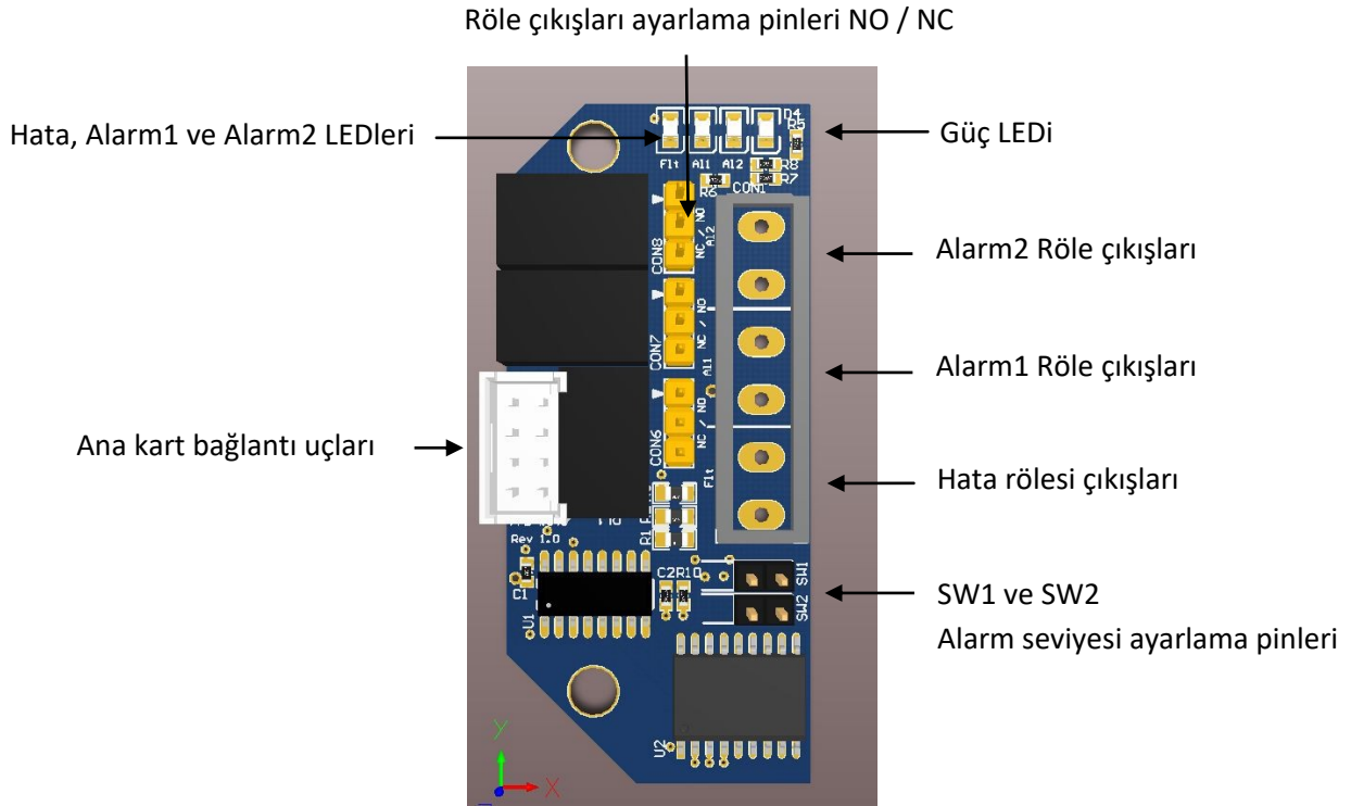
Diagram 9: Röle Modülü
